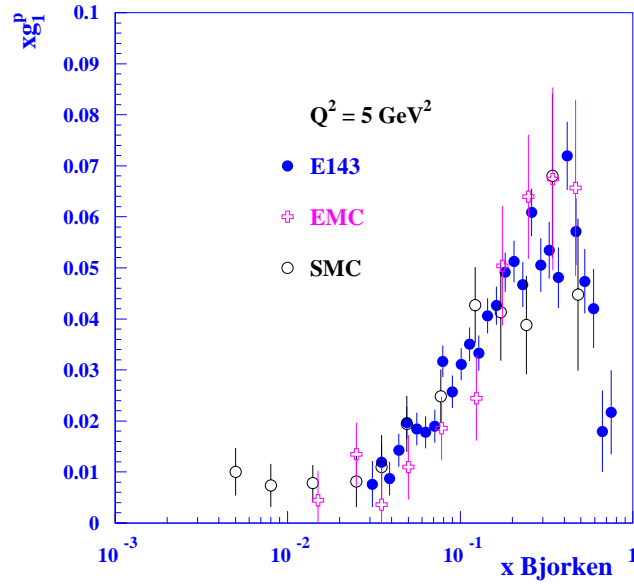
Fig. 2. World data on xg_1^p(x) .
