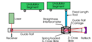
Fig. 4 Interferometer
