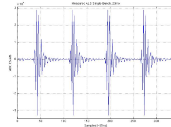
Fig. 1: Measured ALS Single Bunch
