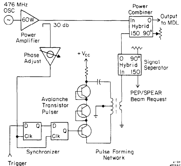
Fig. 3. Fiducial generator.
