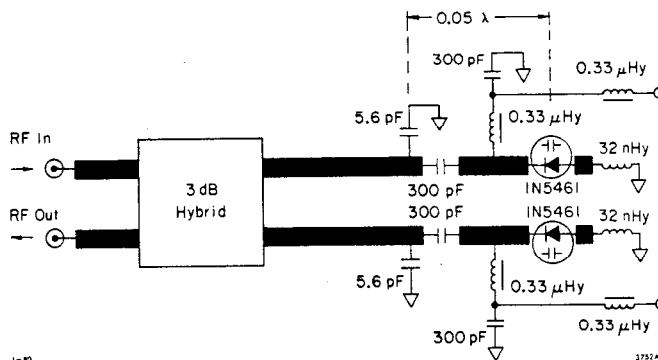
Fig. 6. 180^\circ phase shifter module.
