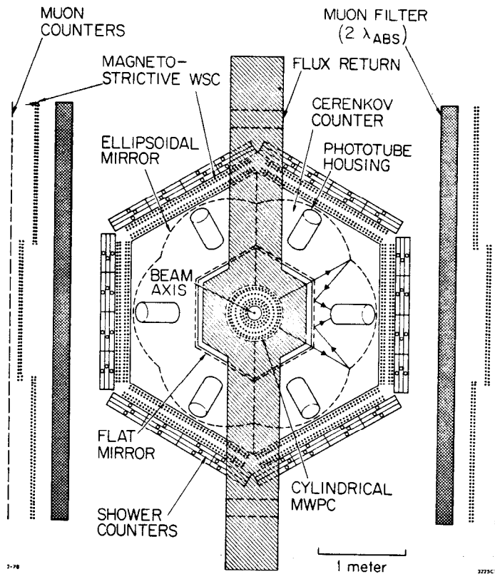
Fig. 1. The DELCO Apparatus
